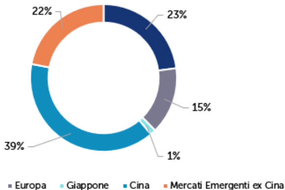
FMI - Contribuzione % alla crescita del PIL 2020
